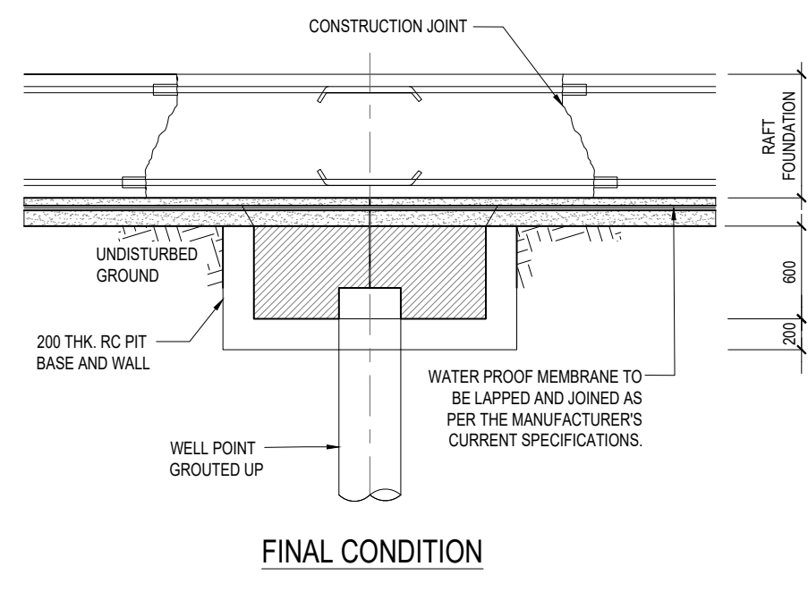
DE-WATERING SUMP IT IN RAFT FOUNDATION SCALE: N.T.S.
